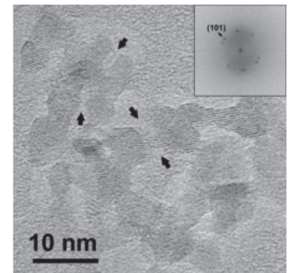
チタニアナノワイヤー。チタニアナノ粒子が、オリエンティッドアタッチメントで、結晶面を揃えて結合し、ネットワーク構造を形成している。
