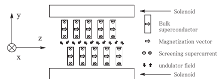
スタガードアレイ型超短周期アンジュレータの概念図
