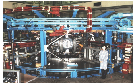
Heliotron J 実験装置
