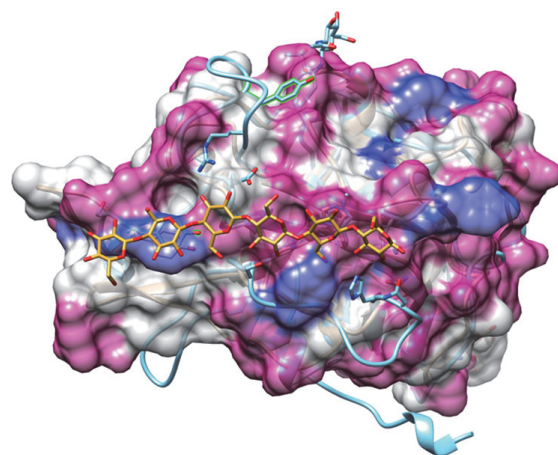
図 1 (左) セルロース (Avicel ないしは PASC) に市販のセルラーゼカクテル (Celluclast 1.5L) を単独で作用させた時と比べ、今回同定した酵素 (CsLPMO) を同時に作用させると、セルロースの分解効率が格段に上昇する。 (右) CsLPMO とセルロースの複合体の構造。この構造に基づいて変異体を作成したところ、分解効率のさらなる向上が達成された (ACS Sustain. Chem. Eng., 9, 16651, 2022 より引用／改変)。
