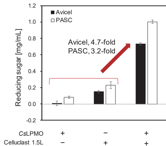
図 1 (左) セルロース (Avicel ないしは PASC) に市販のセルラーゼカクテル (Celluclast 1.5L) を単独で作用させた時と比べ、今回同定した酵素 (CsLPMO) を同時に作用させると、セルロースの分解効率が格段に上昇する。 (右) CsLPMO とセルロースの複合体の構造。この構造に基づいて変異体を作成したところ、分解効率のさらなる向上が達成された (ACS Sustain. Chem. Eng., 9, 16651, 2022 より引用／改変)。
