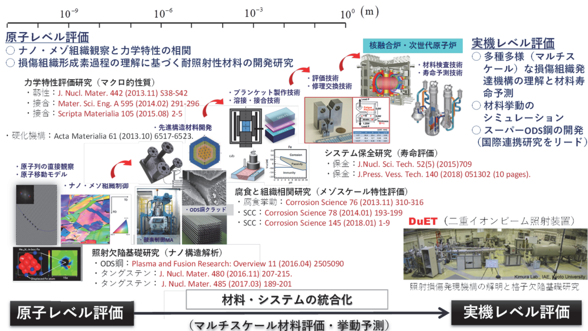
図1 原子炉材料の保全と革新的原子炉構造材料の開発に向けたエネルギー基盤材料の照射損傷形成機構解明のための材料挙動マルチスケール・マルチフィジクス解析手法
