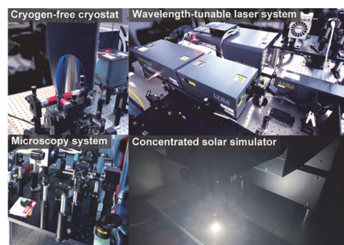
図2 エネルギー機能物性計測設備群
