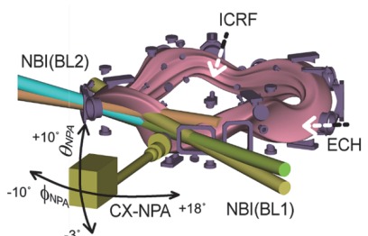
3 ヘリオトロン J 用中性粒子ビーム入射加熱装置概要図
