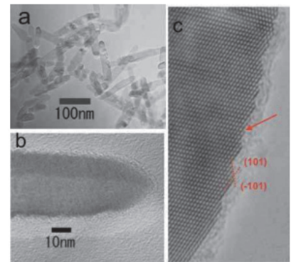
チタニアナノロッドの TEM 像。その高分解能像では、チタニア原子が結晶面にきれいに整理している。また、その表面に色素分子が吸着しているのわかる。
