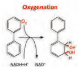
C. BDOがビフェニルへ酸素を添加し、一方の芳香環を水酸化する酵素反応。
