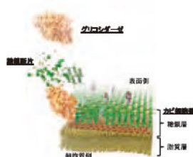
F. グリコシダーゼがカビの細胞壁を消化する様子を表したイメージ。
