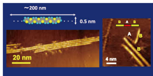
導電性高分子の1分子細線
