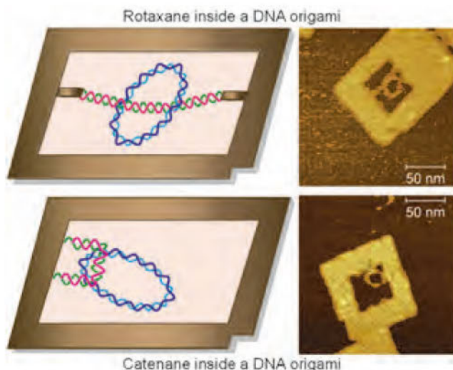
DNA オリガミフレーム内に構築されたロタキサン構造
